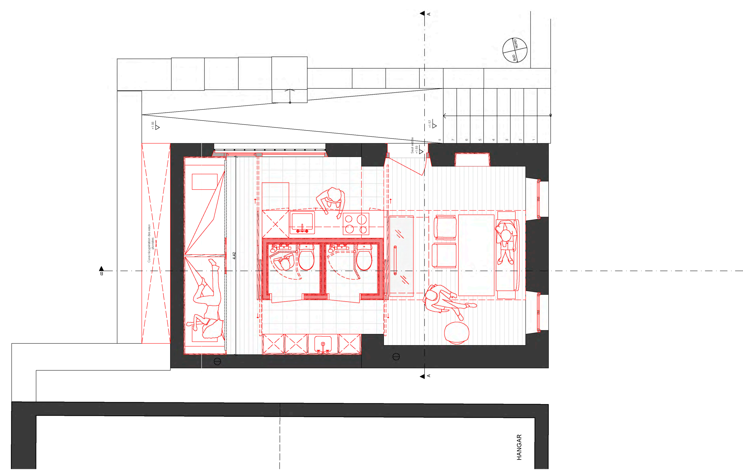
Premier étage
