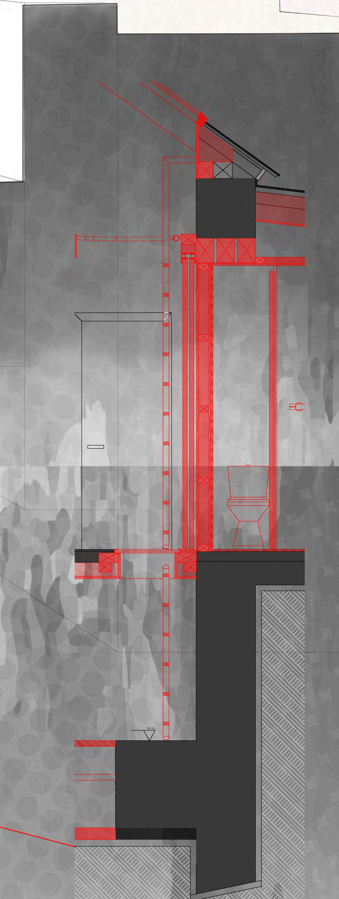
Détail 1:20
