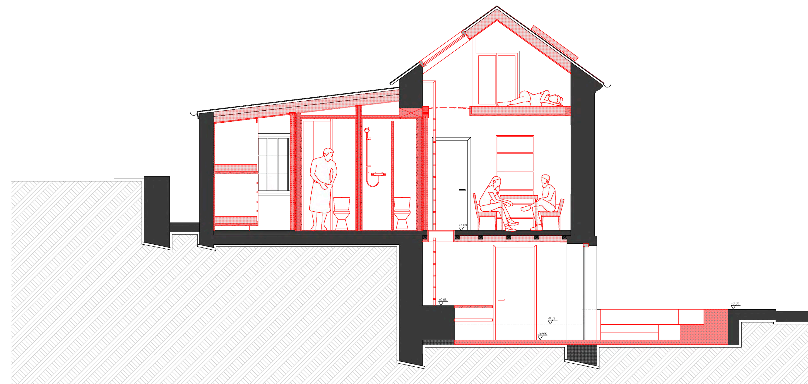
Coupe B
